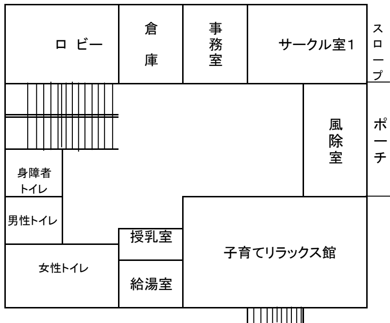
（1階平面図）
